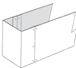
1 En U boulonné avec plaques arrières
